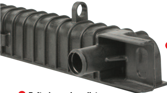
2 Boîte à eau de radiateur
